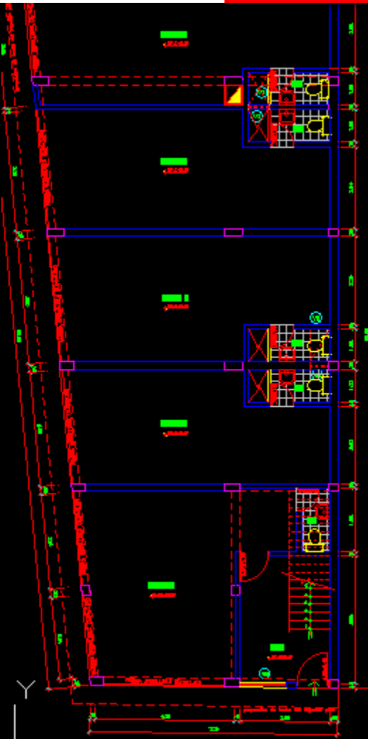
PLANTA PRIMER PISO Esc. 1/30
