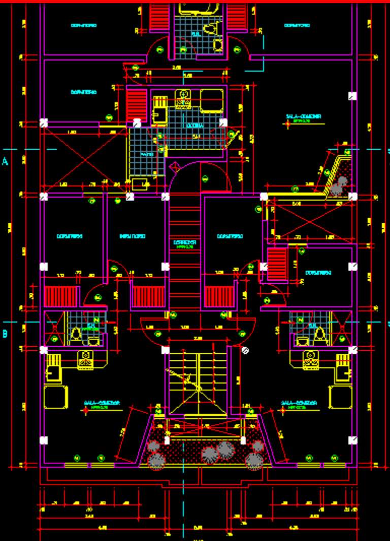
SEGUNDO PISO
