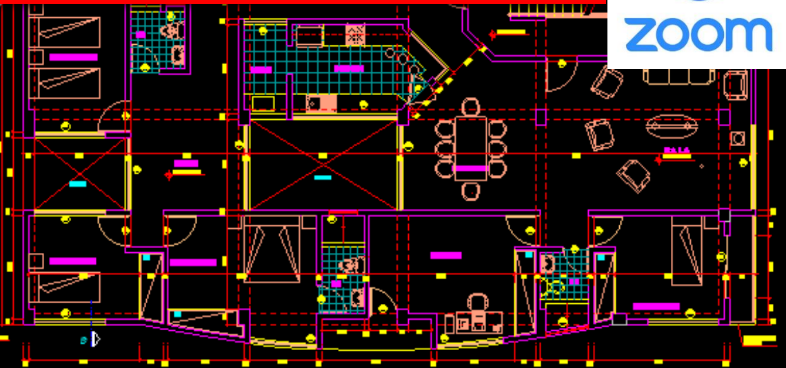
PLANTA: SEGUNDO PISO Esc: 1/80
