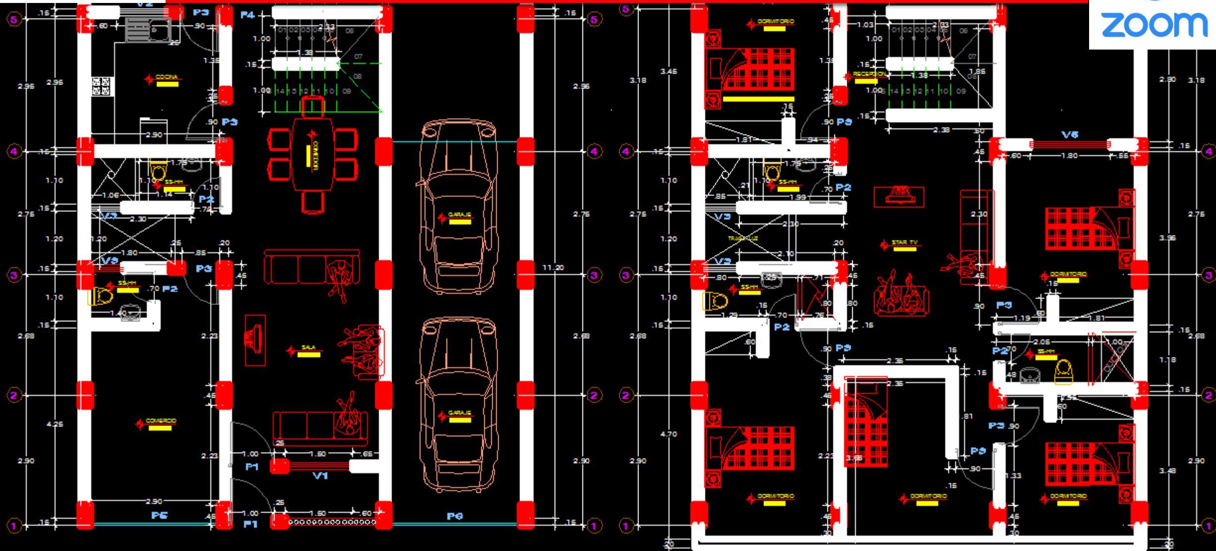
1° NIVEL ESC: 1/50
