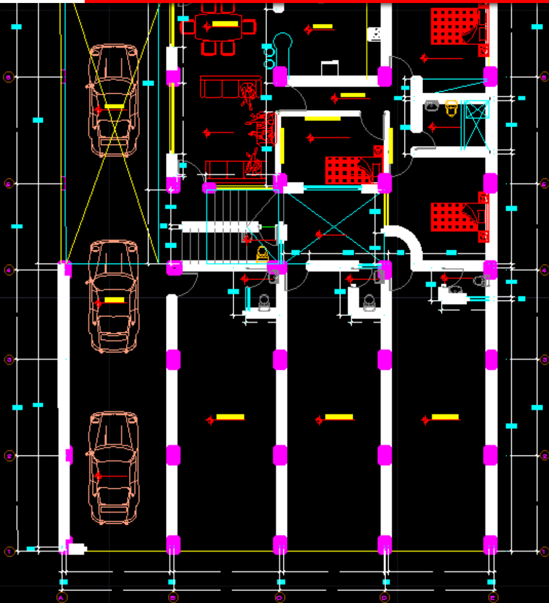
1º NIVEL DISTRIBUCION
