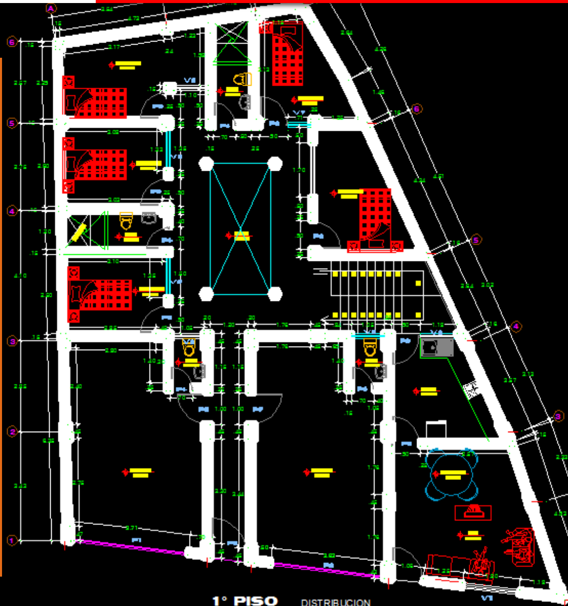
1° PISO DISTRIBUCION ESC: 1/50
