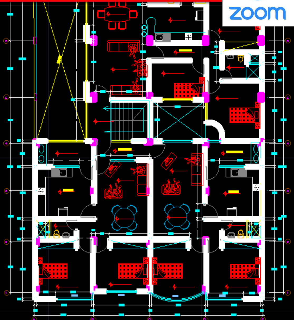
2º NIVEL DISTRIBUCION
