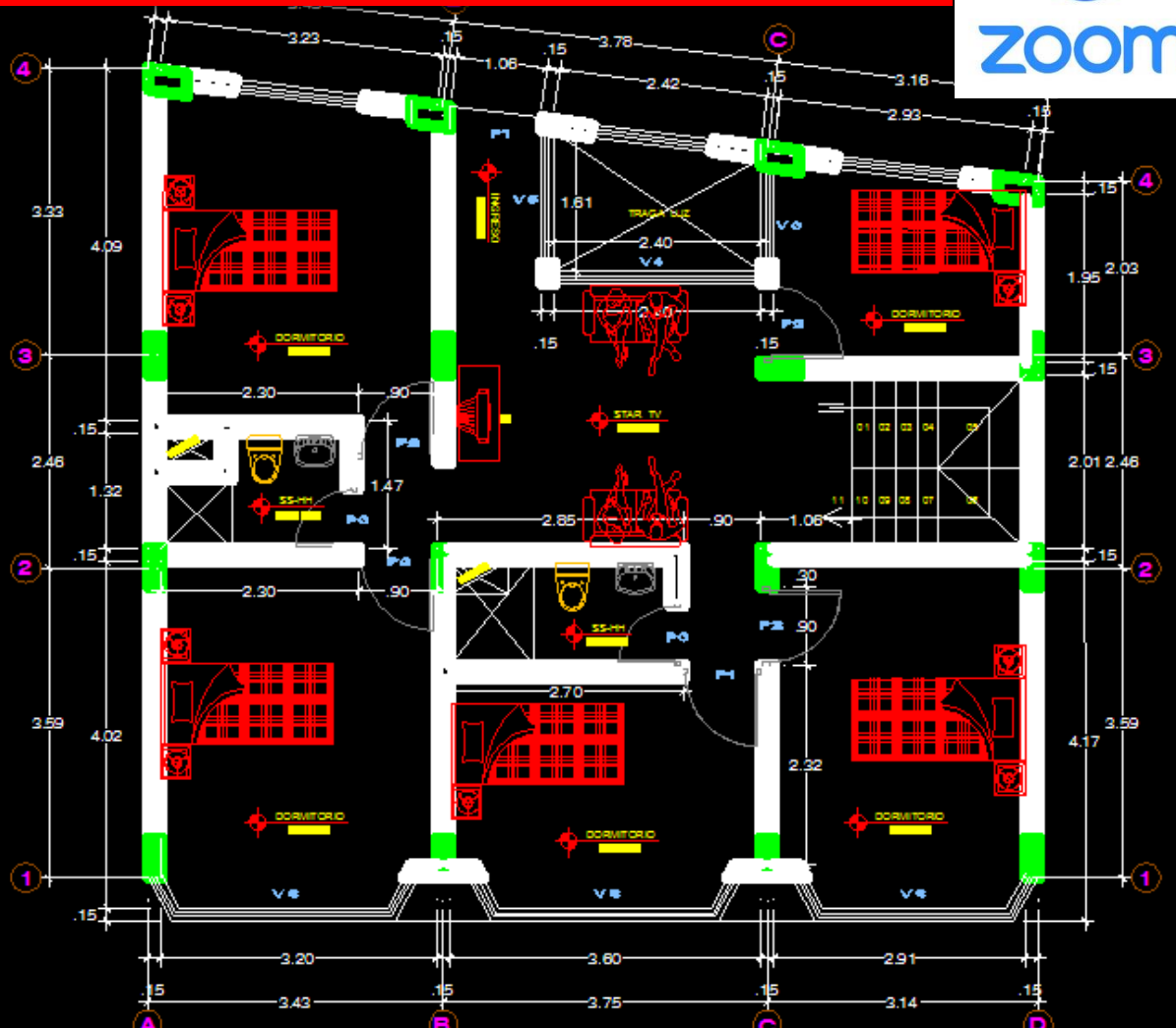
2º NIVEL DISTRIBUCION ESC: 1/50
