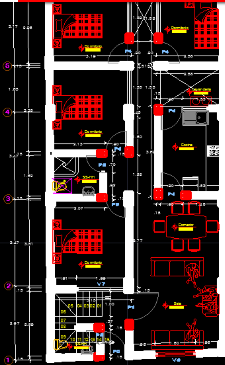
1º NIVEL ESC: 1/50 DISTRIBUCION
