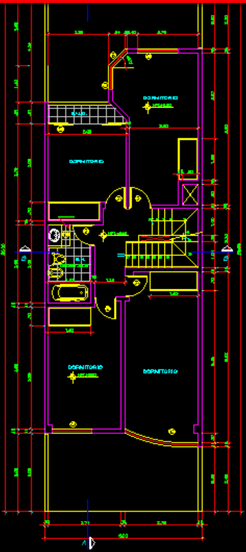
SEGUNDO ESC. 1/50
