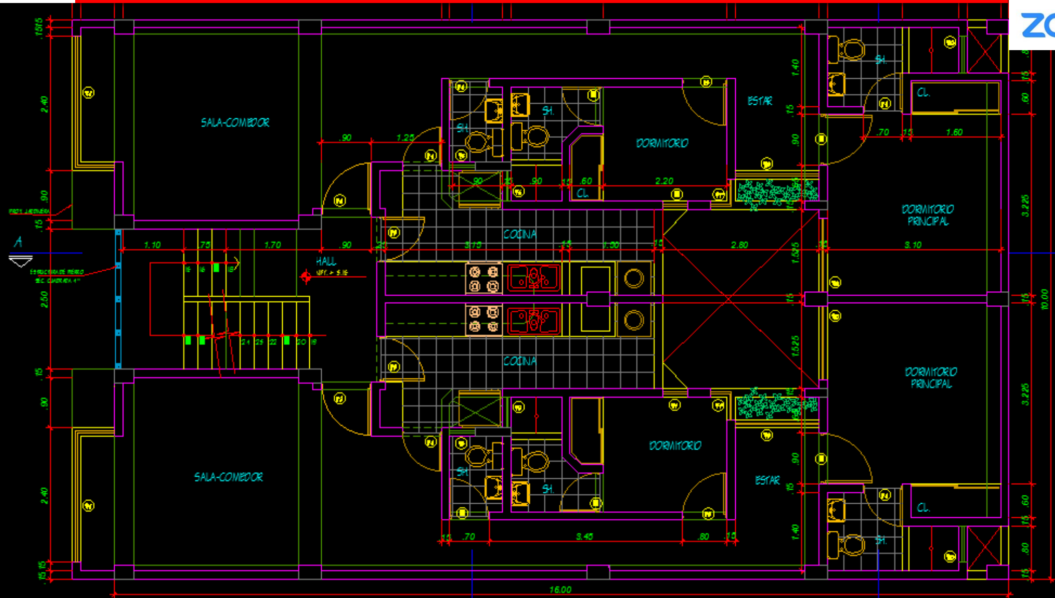
PLANTA: SEGUNDO PISO
