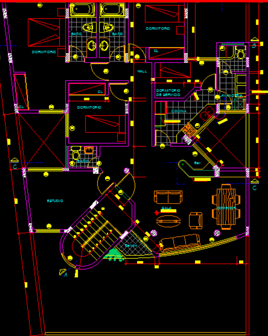
PLANTA: SEGUNDO PISO PLANTA: SEGUNDO PISO
