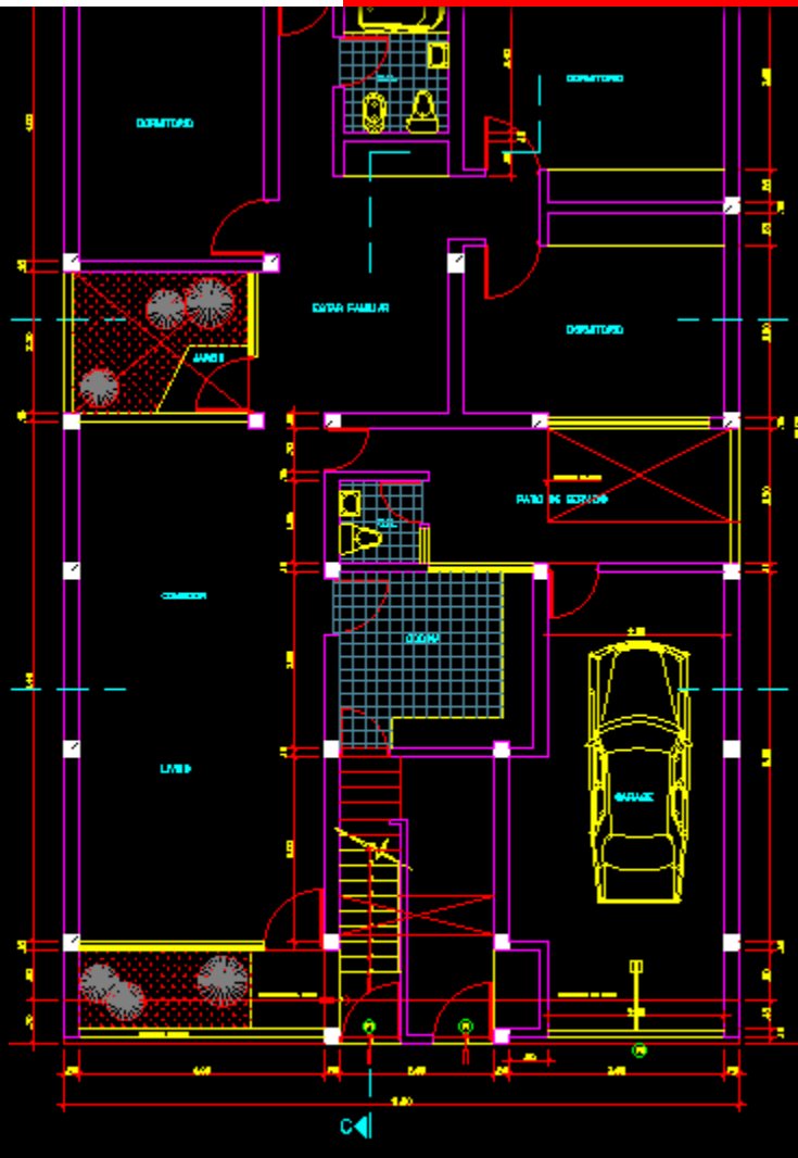
PRIMER PISO ESCALA: 1 / 50
