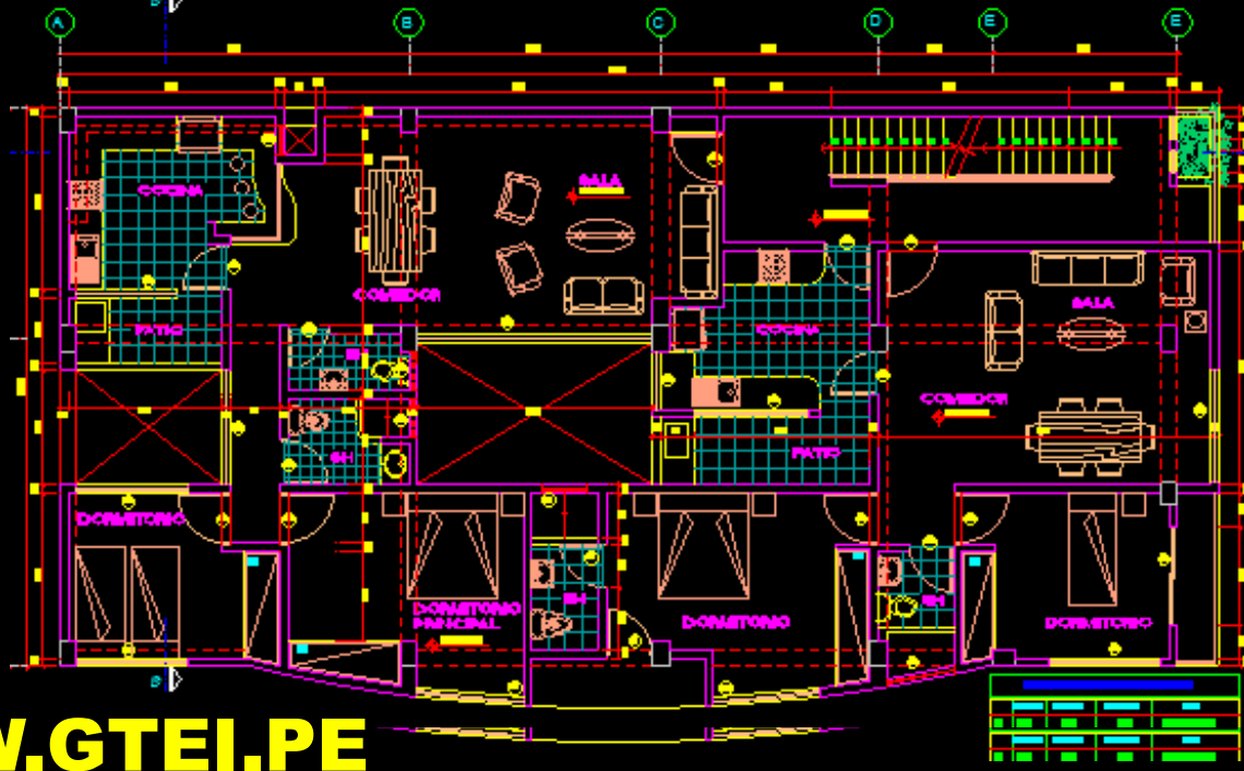
PLANTA: PRIMER PISO Esc: 1/80
