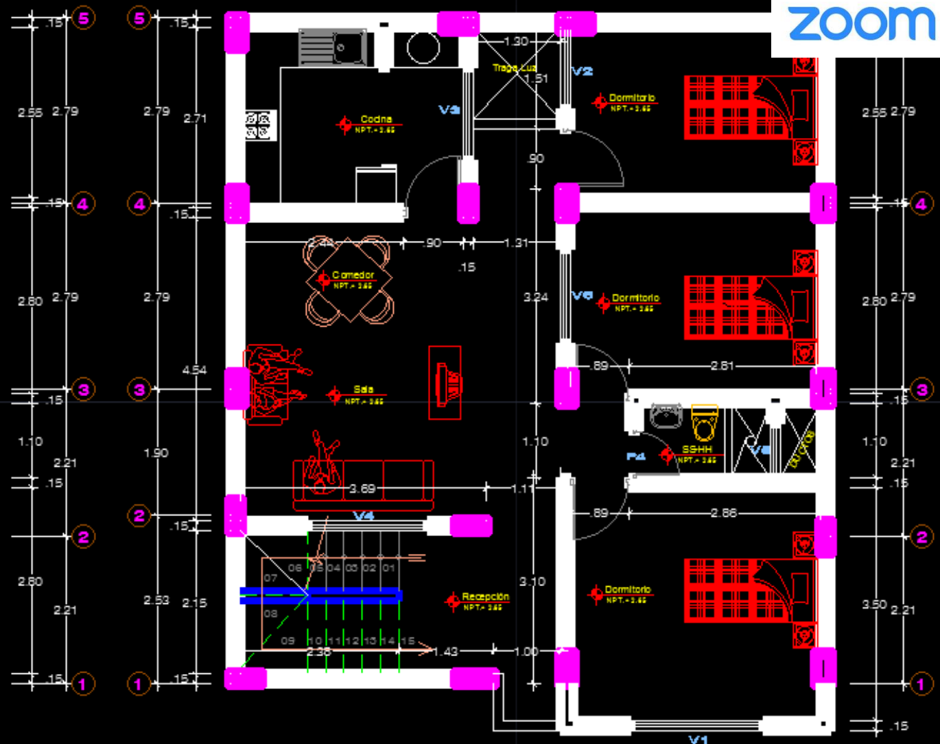
2° NIVEL ESC: 1/50
