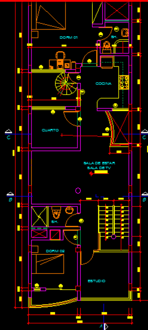
PLANTA: TERCER PISO ESC. 1/50
