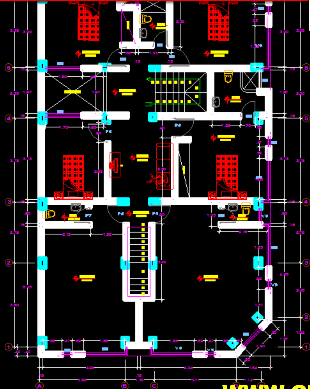
2º NIVEL DISTRIBUCION
