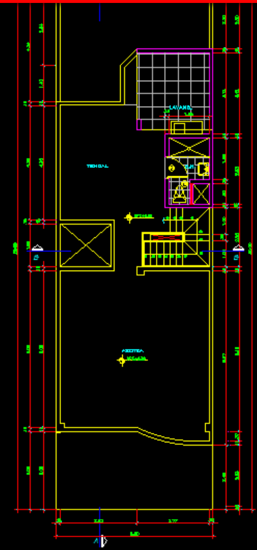
TERCERO ESC. 1/50
