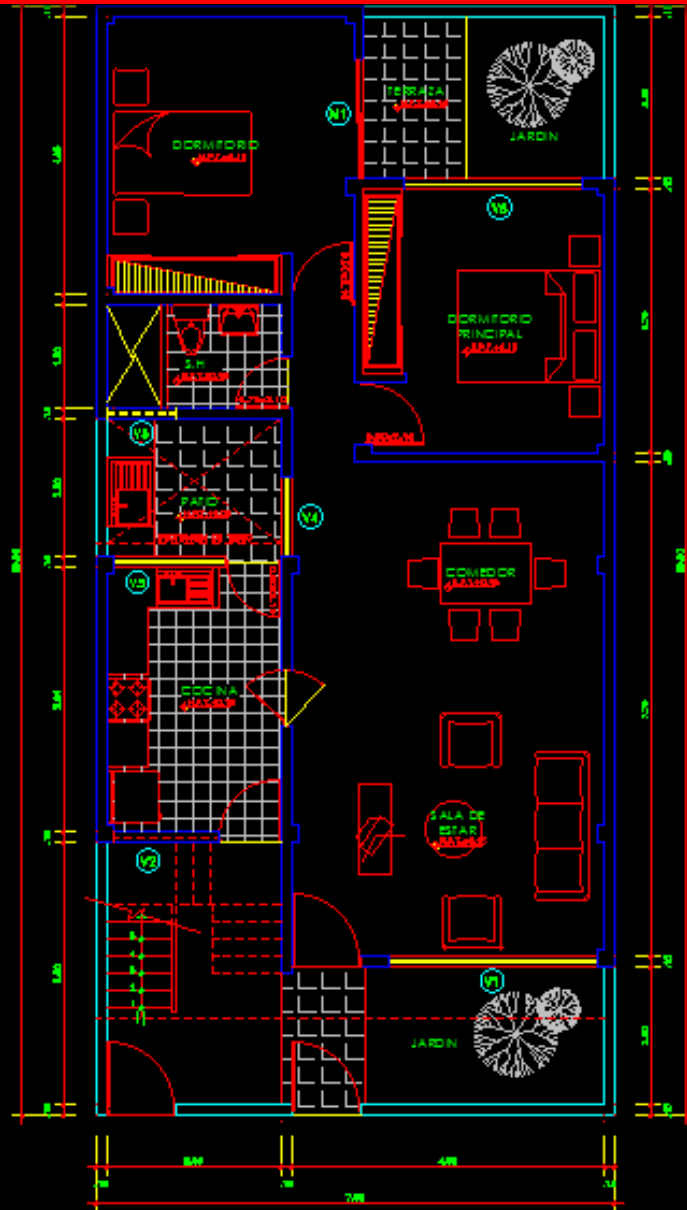
PLANTA PRIMER PISO
