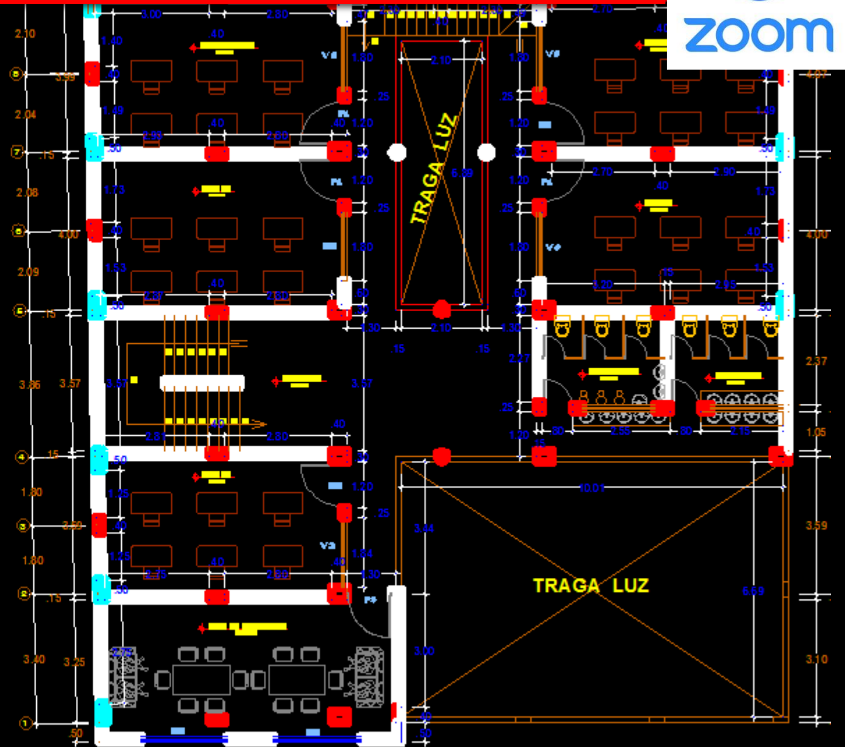
2° NIVEL ESC: 1/50
