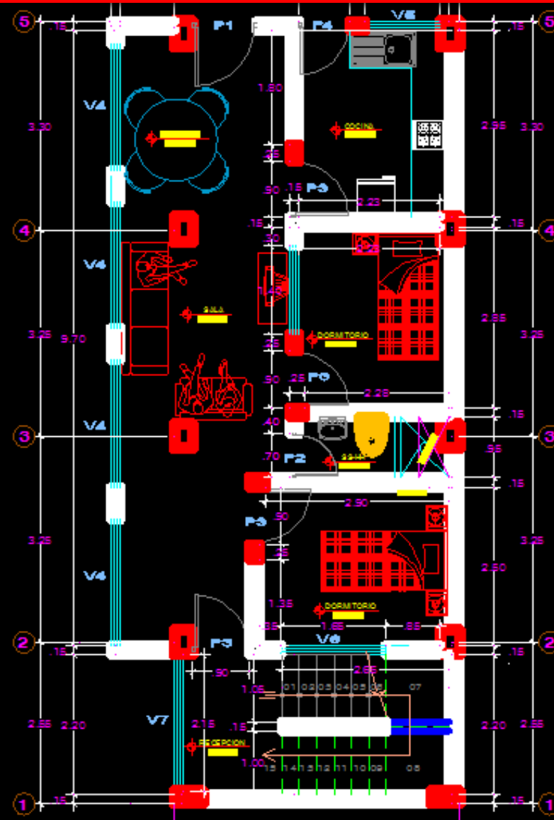
2º NIVEL
