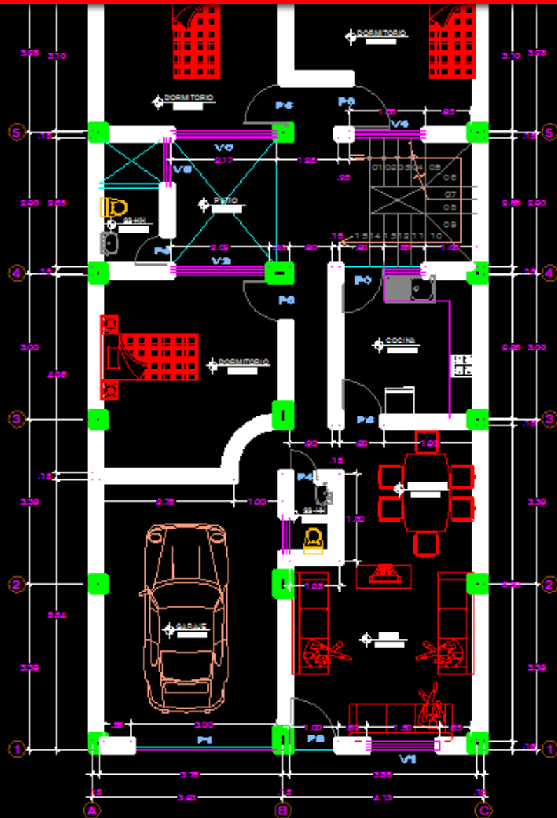
1er NIVEL ESC: 1/50
