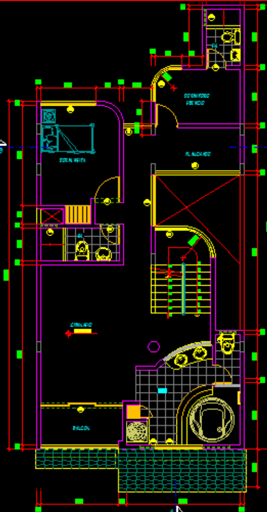
PLANTA: TERCER PISO ESC. 1/50
