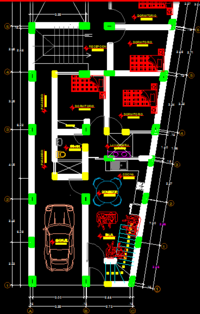
2º NIVEL Distribución ESC: 1/50
