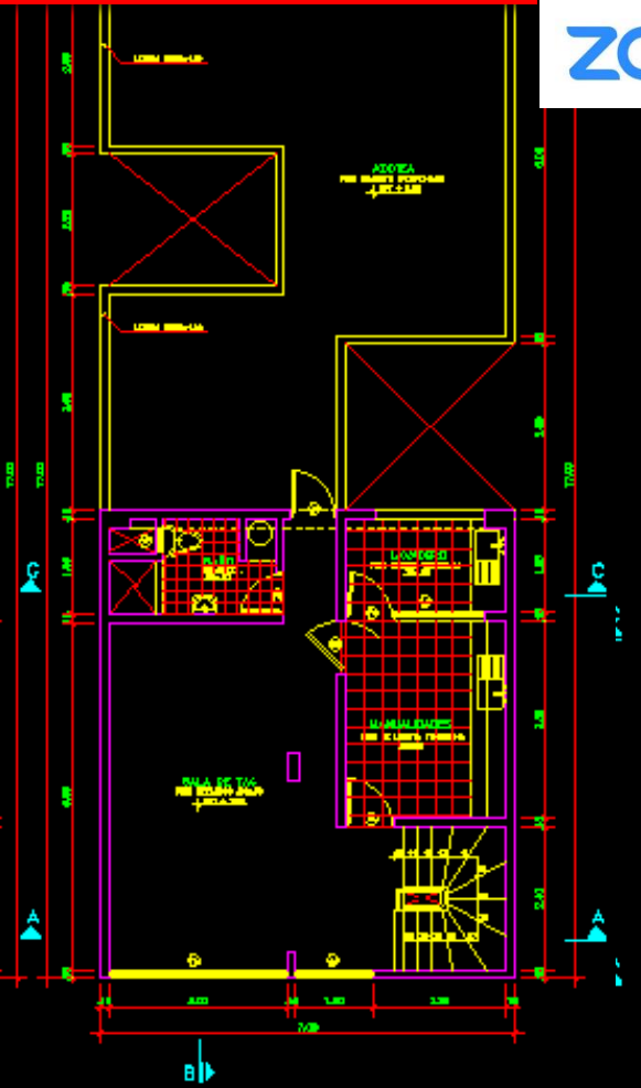
TERCERA PLANTA ESCALA : 1/50
