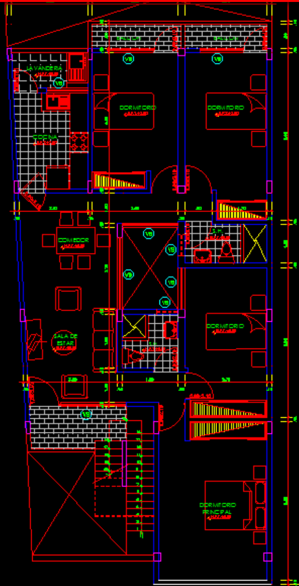
PLANTA SEGUNDO PISO
