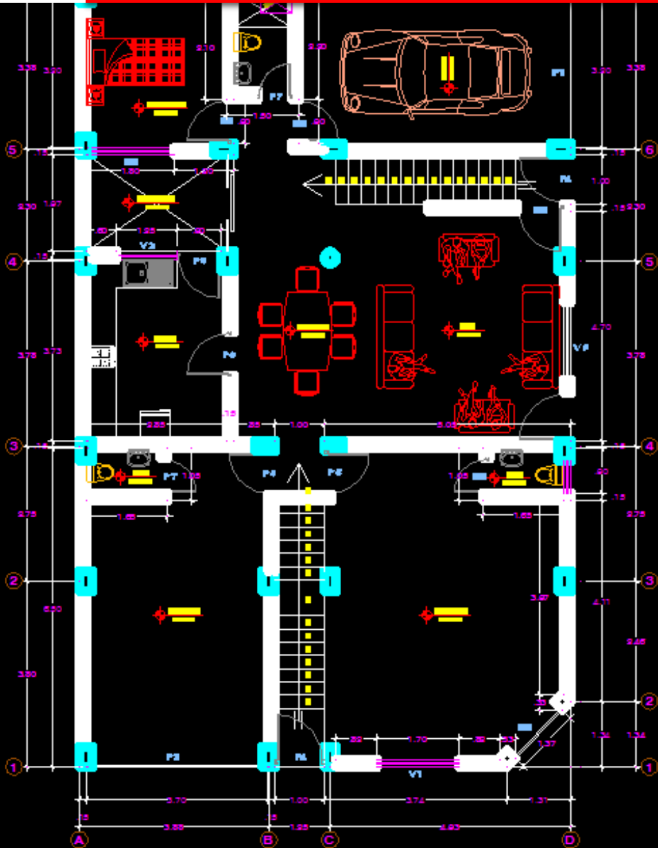
1º NIVEL DISTRIBUCION
