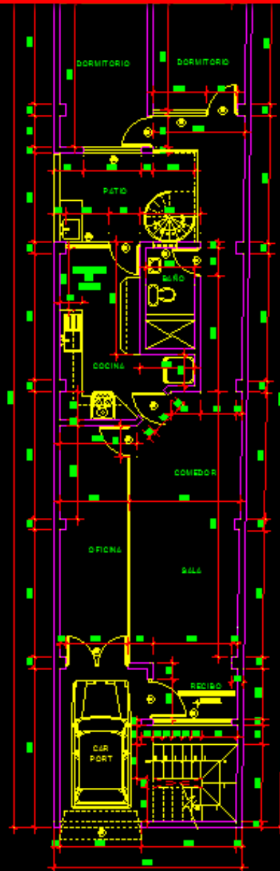
PRIMER PISO
