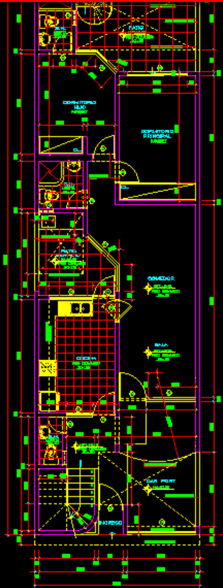
PLANTA PRIMER PISO ESC. 1/80
