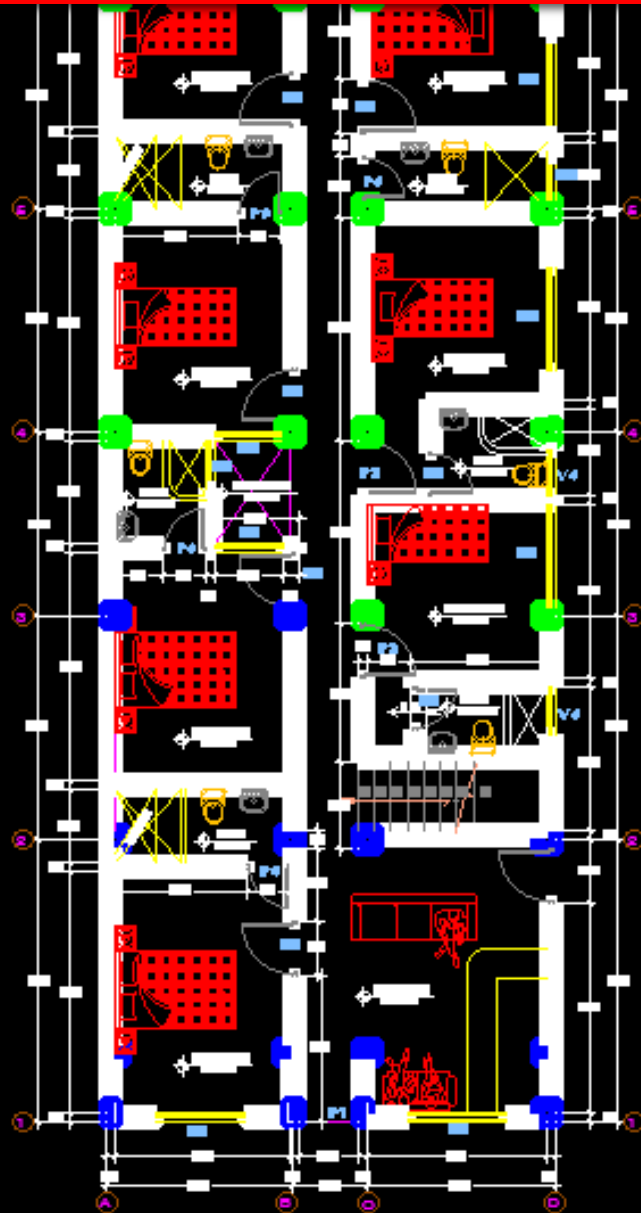
1er NIVEL ESC: 1/50 DISTRIBUCION
