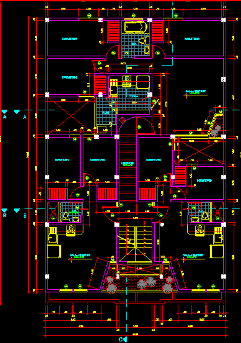
SEGUNDO PISO ESCALA: 1 / 50
