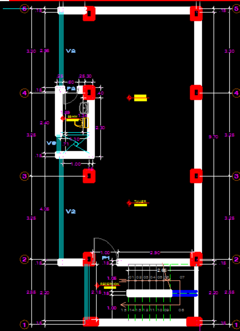
1º NIVEL
