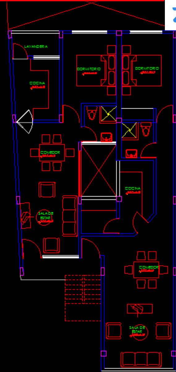
PLANTA TERCER PISO
