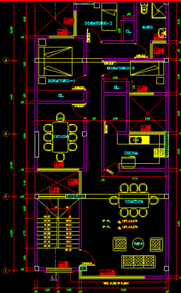
2ª / 3ª PLANTA
