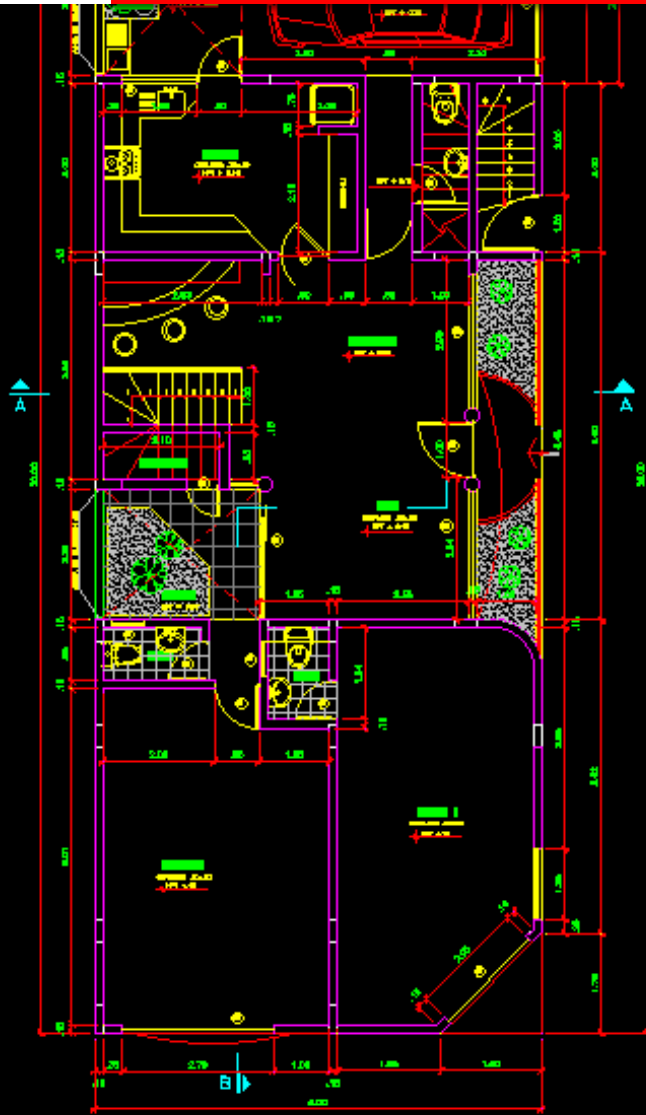
PRIMER PISO
