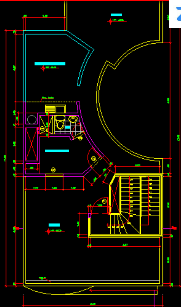
PLANTA AZOTEA ESC. 1/50
