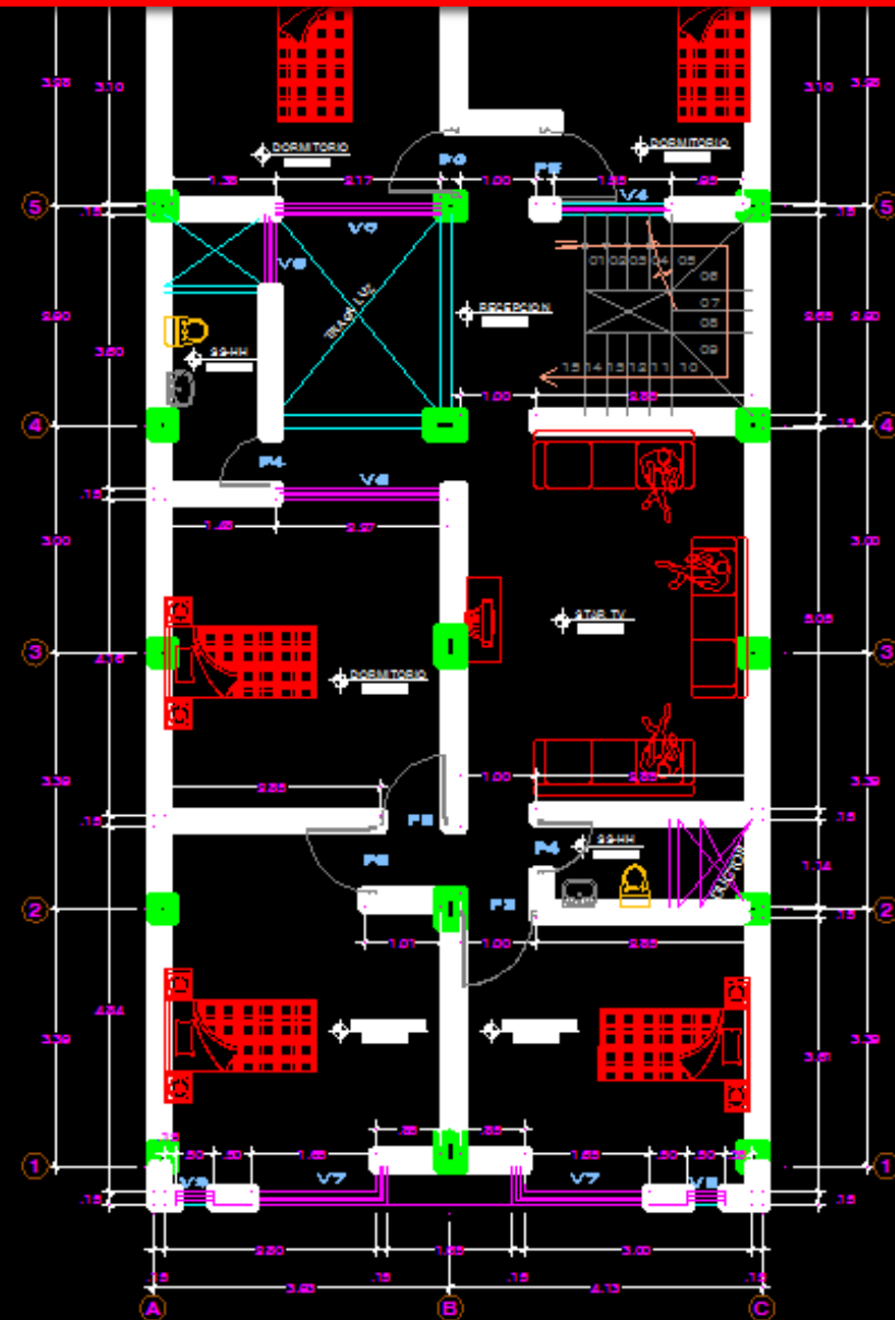
2er NIVEL ESC: 1/50
