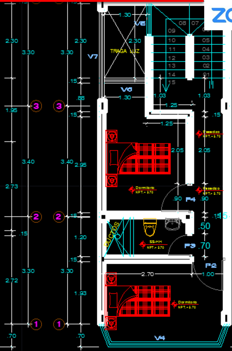
3º NIVEL DISTRIBUCION ESC: 1/50
