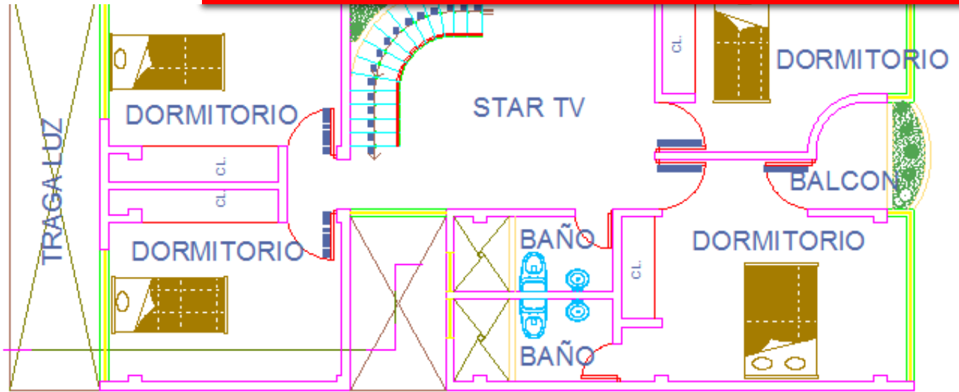
SEGUNDO PISO
