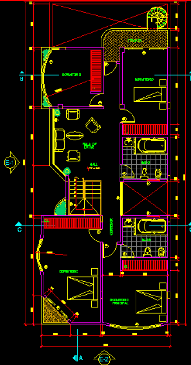
SEGUNDO PISO
