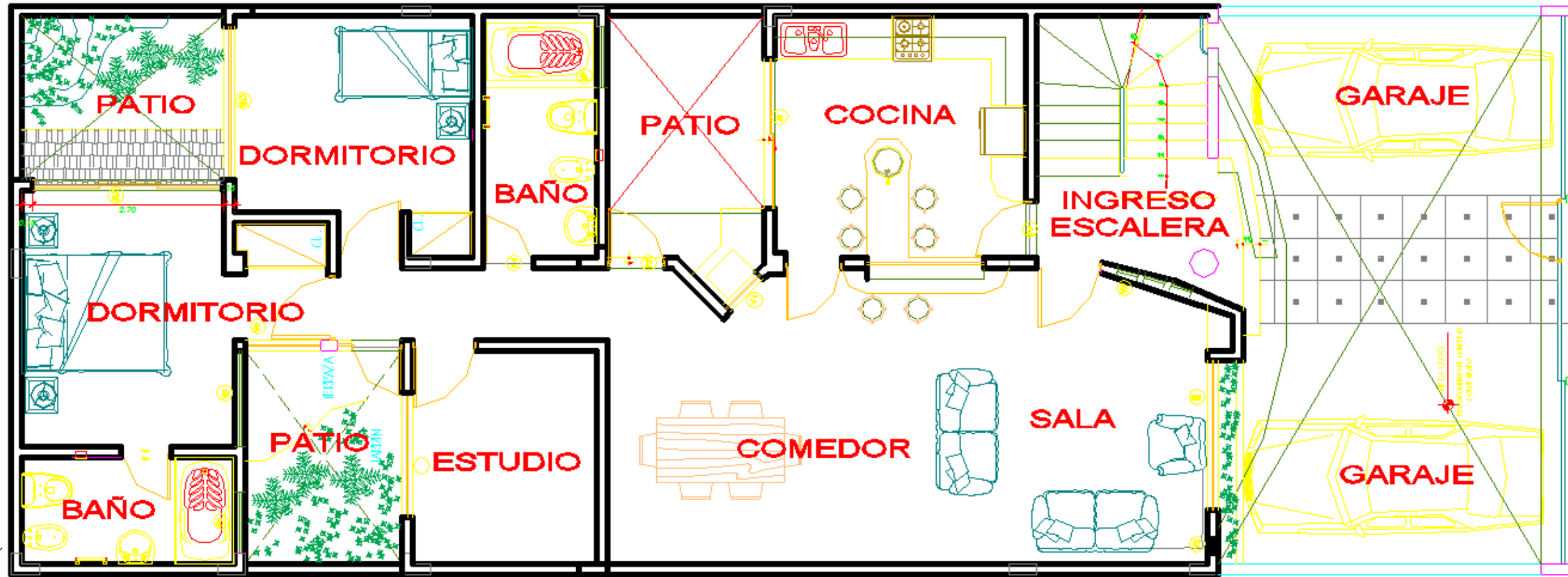
PLANTA: PRIMER PISO
