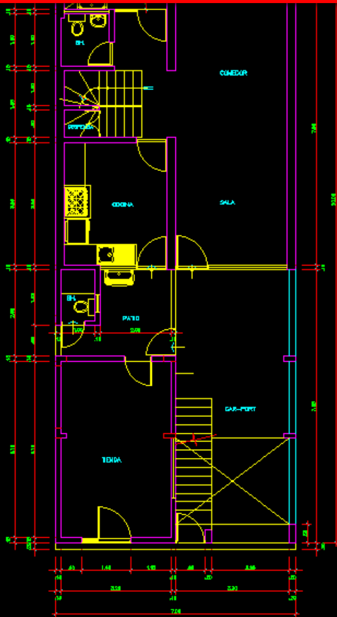
PRIMER PISO ESCALA 1/50
