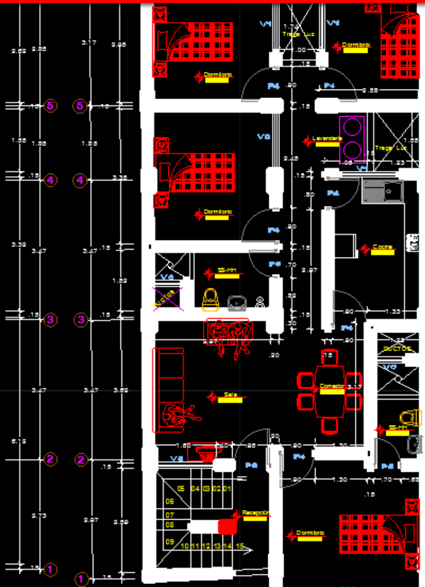
2º NIVEL ESC: 1/50 DISTRIBUCION
