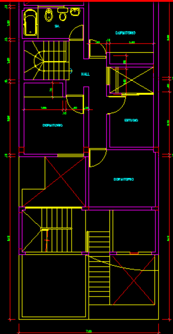
SEGUNDO PISO ESCALA 1/50
