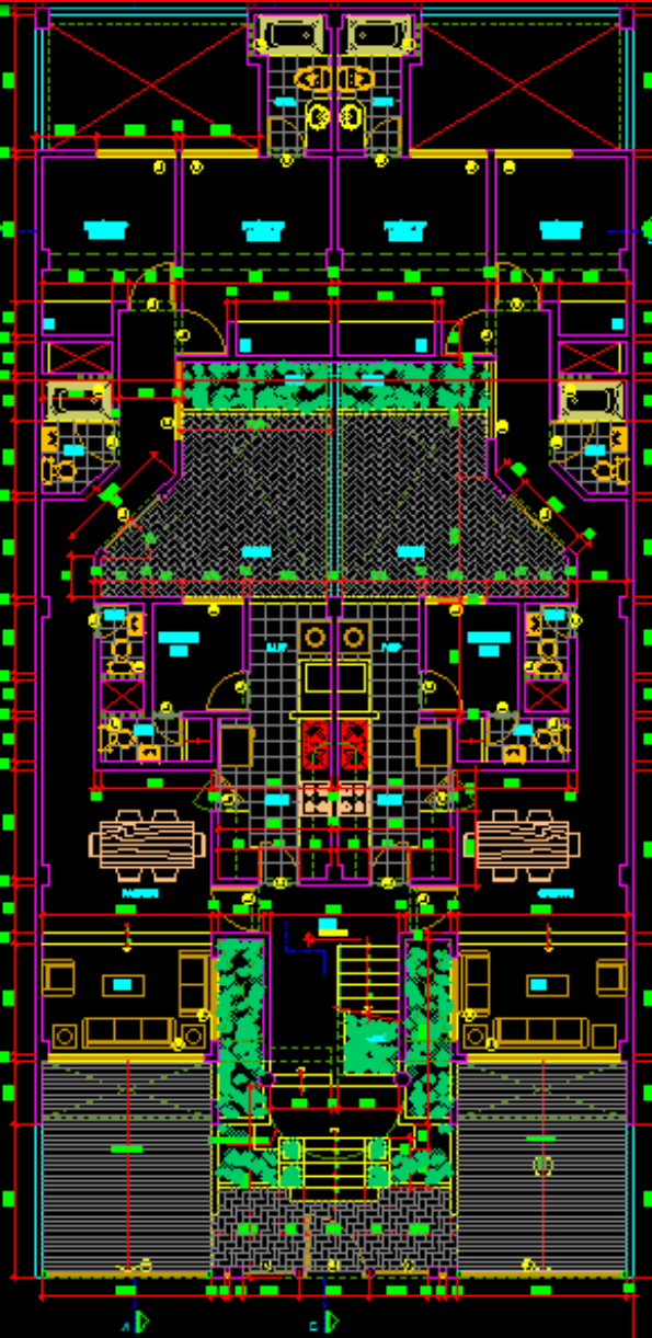
PLANTA: PRIMER PISO ESC. 1/50
