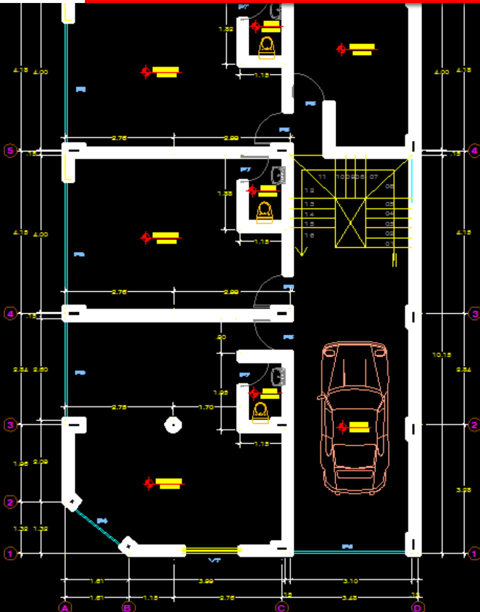
1º NIVEL DISTRIBUCION ESC 1:50
