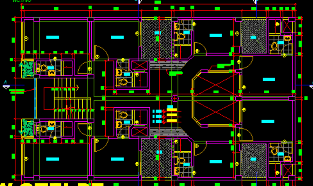
PLANTA: PRIMER PISO ESC. 1/50
