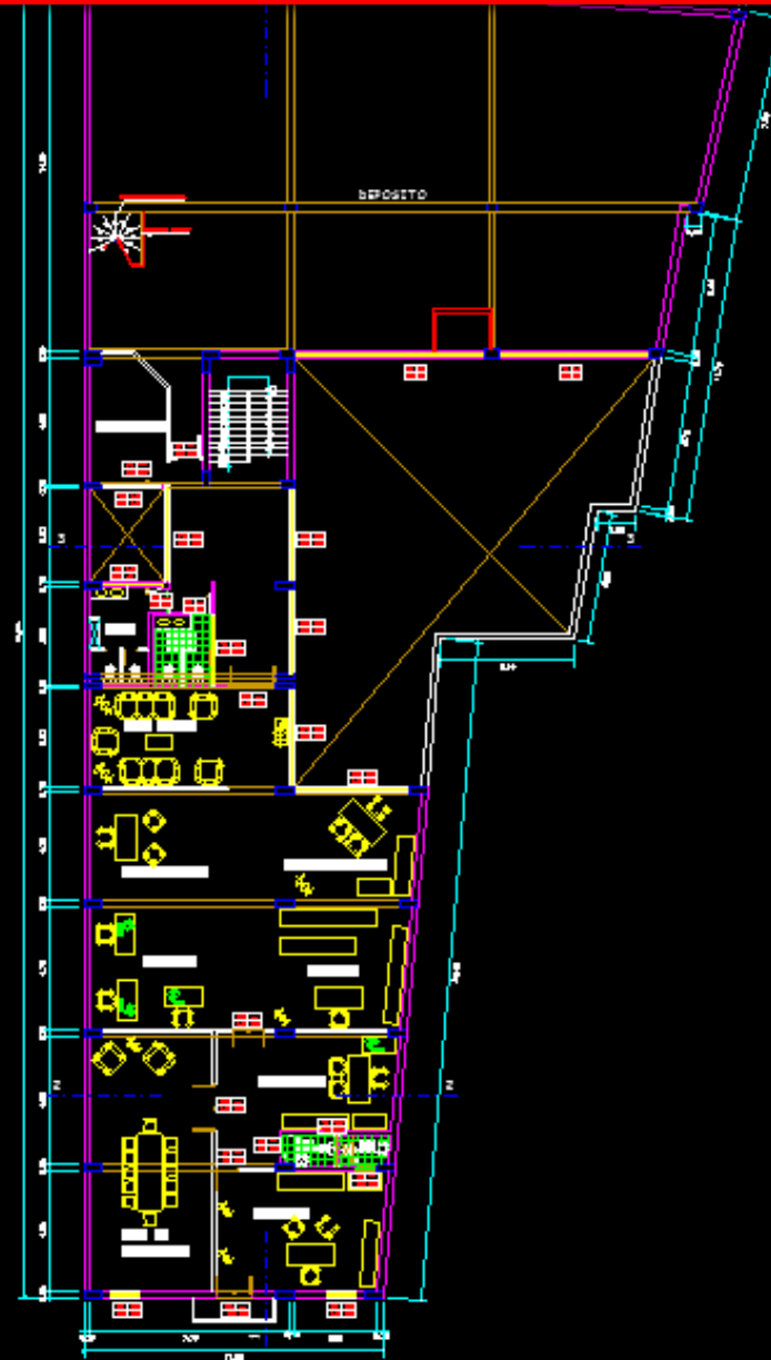
PLANTA SEGUNDO PISO
