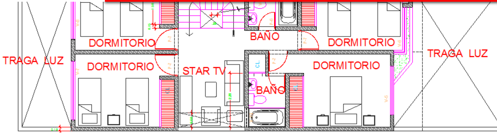
SEGUNDO PISO
