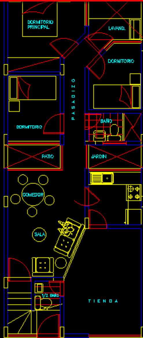
PRIMER PISO ESQ. 1/100
