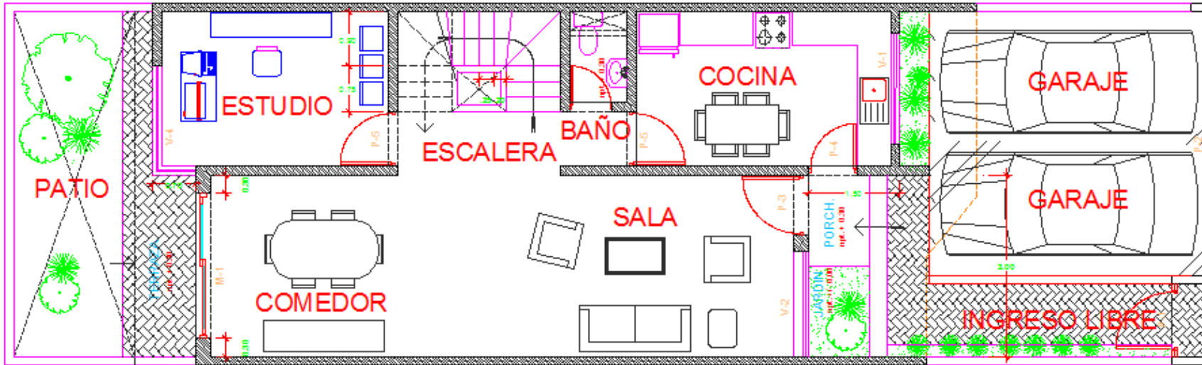
PRIMER PISO
