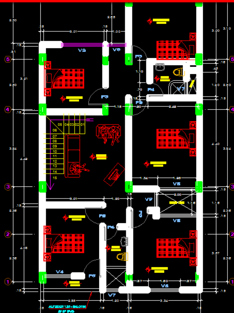
2º NIVEL DISTRIBUCION E.S.C. 1/50
