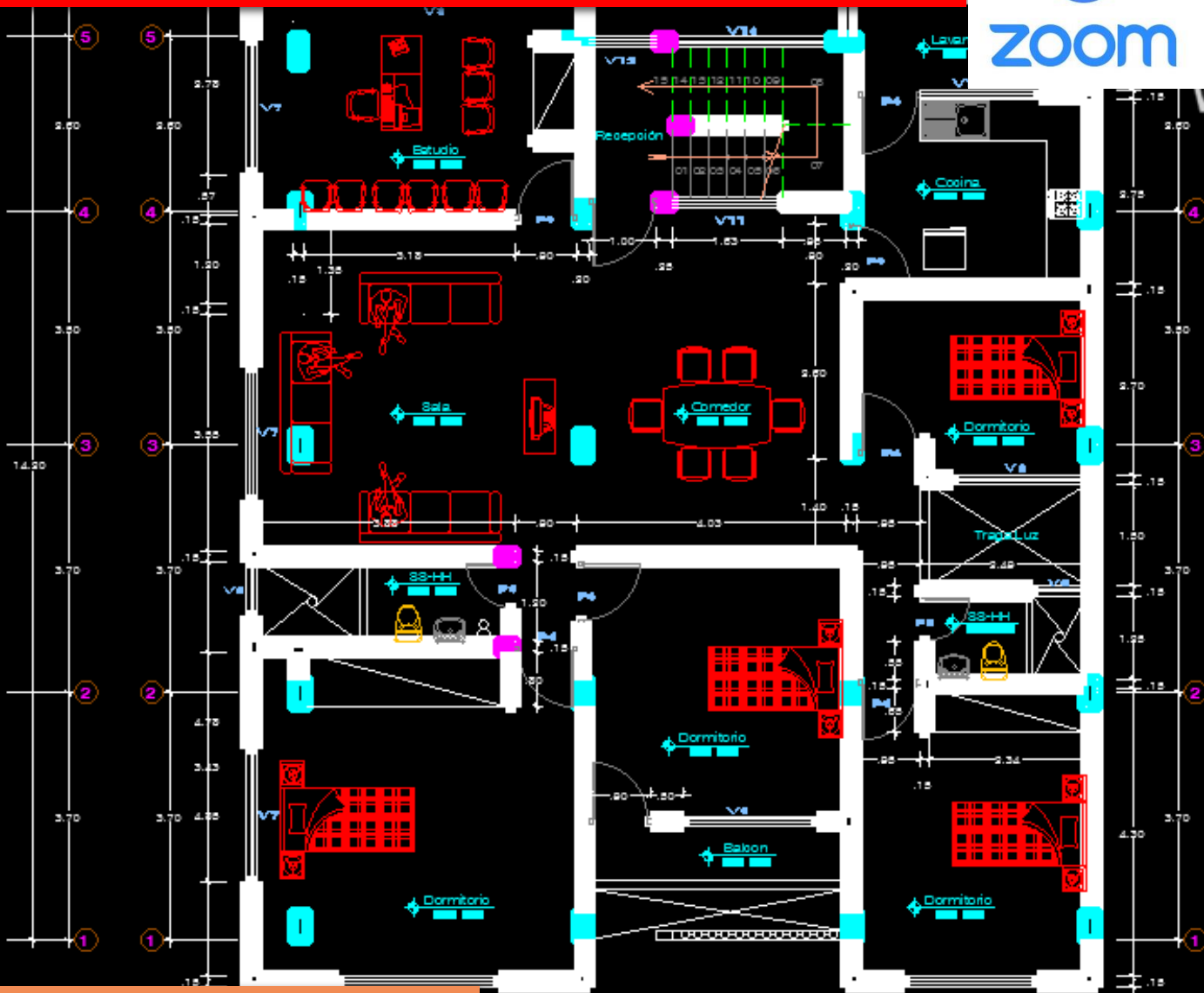
2º NIVEL DISTRIBUCION ESC: 1/50
