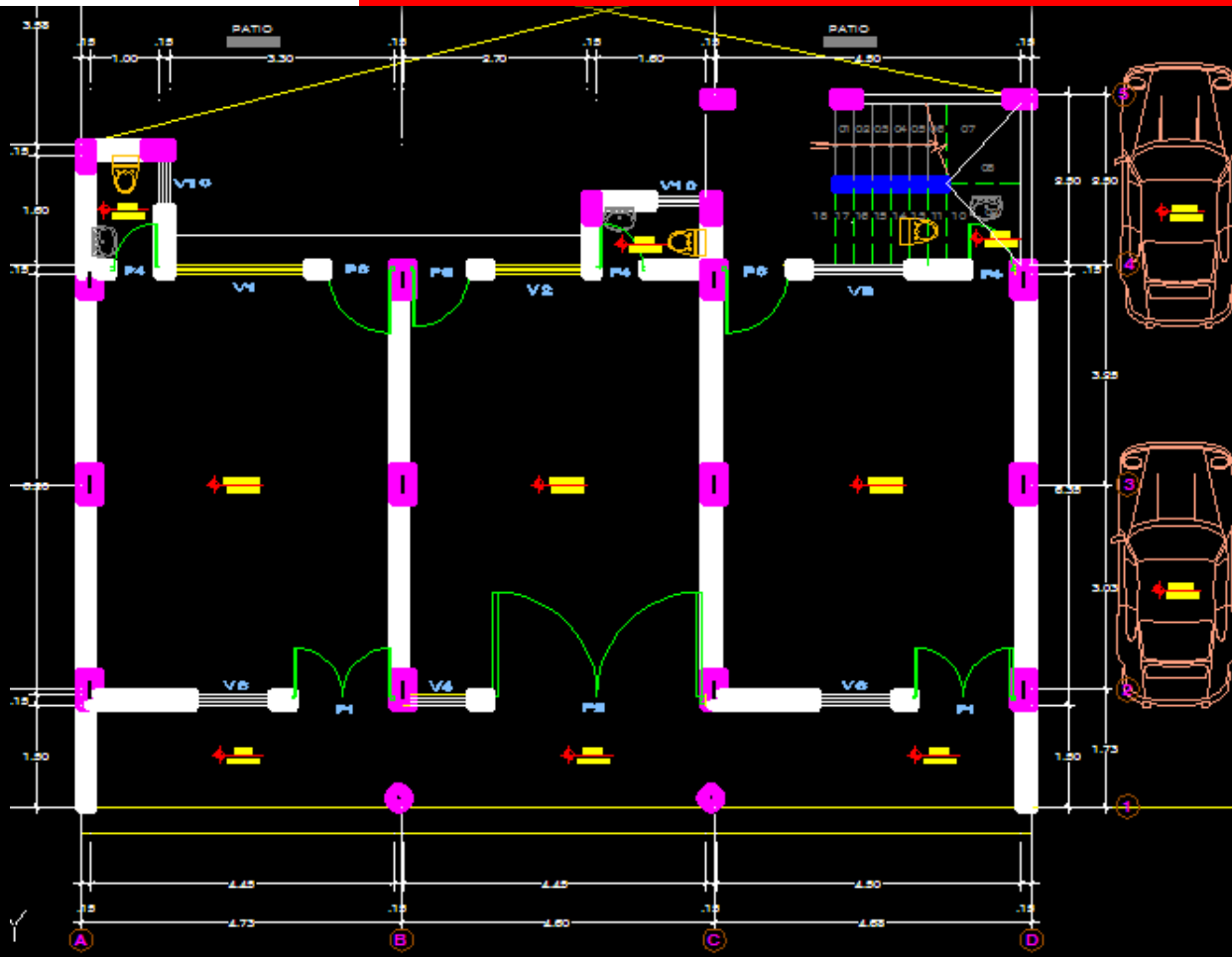
1° NIVEL DISTRIBUCION E.S.C. 1:50
