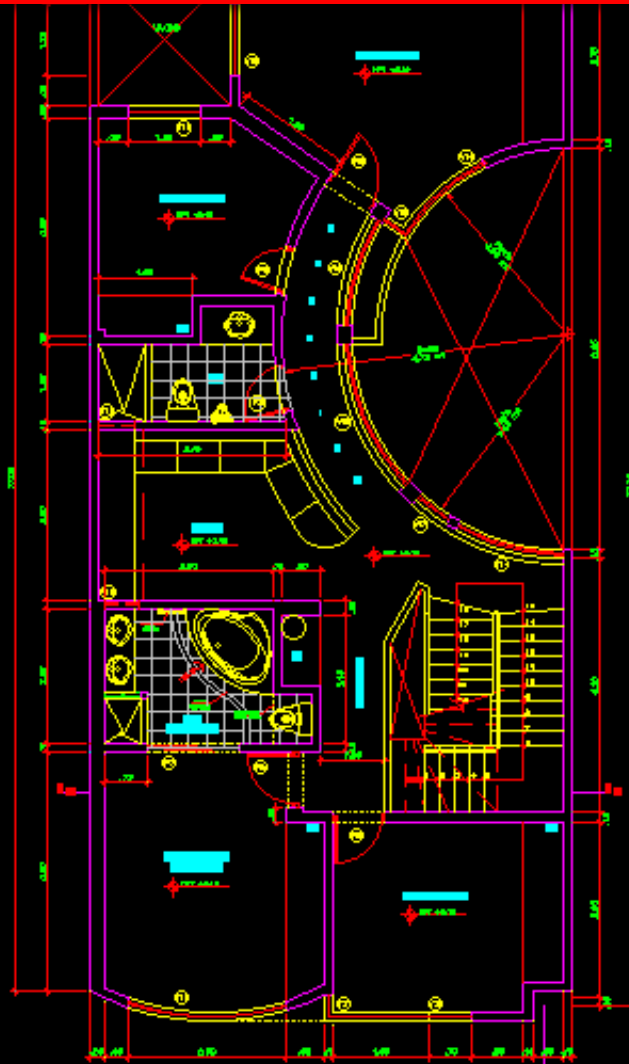
PLANTA SEGUNDO PISO ESC. 1/50
