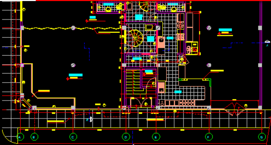
PLANTA: PRIMER PISO ESC. 1/50
