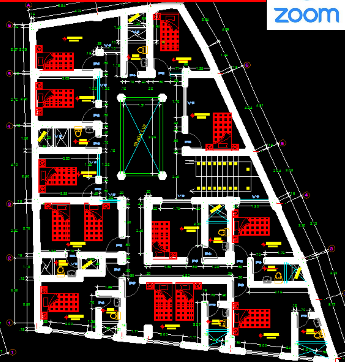
2° PISO DISTRIBUCION ESC: 1/50
