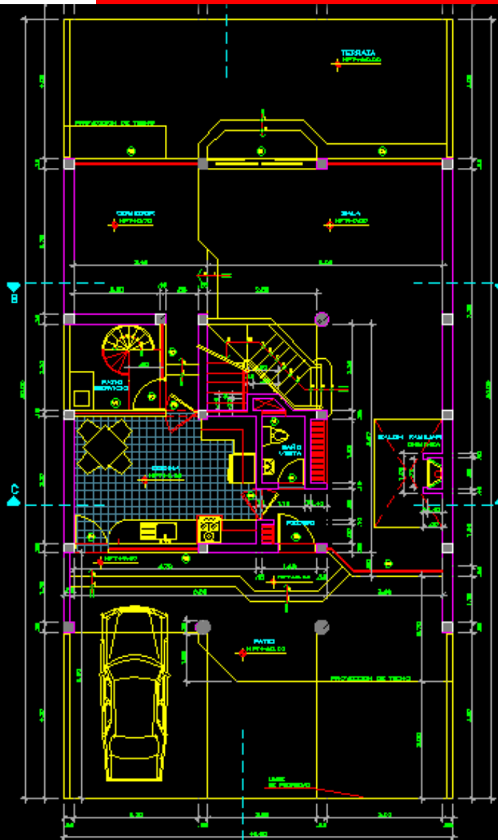
PRIMER PISO
