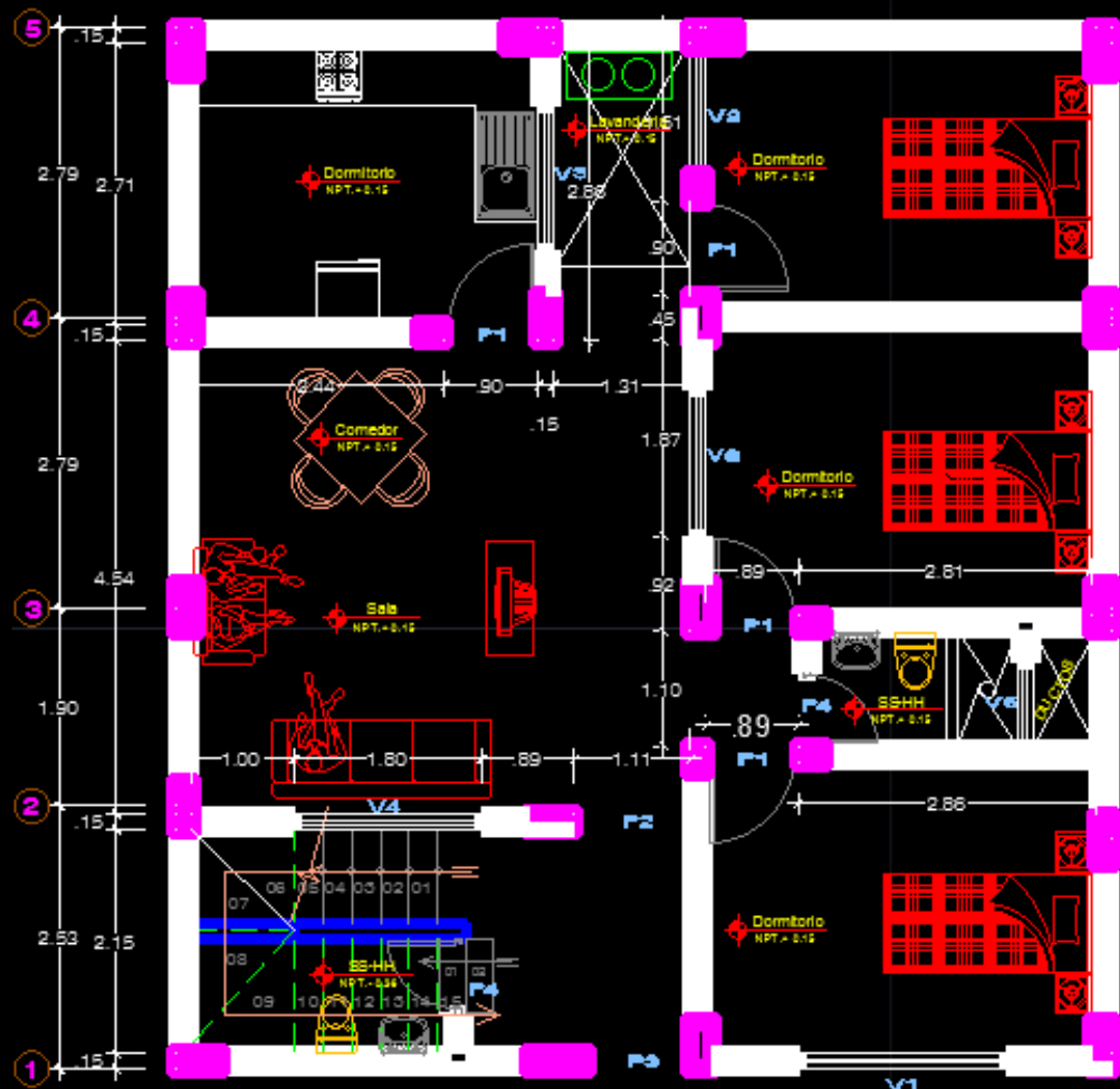
1° NIVEL ESC: 1/50
