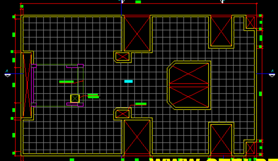
PLANTA: SEGUNDO PISO ESC. 1/50
