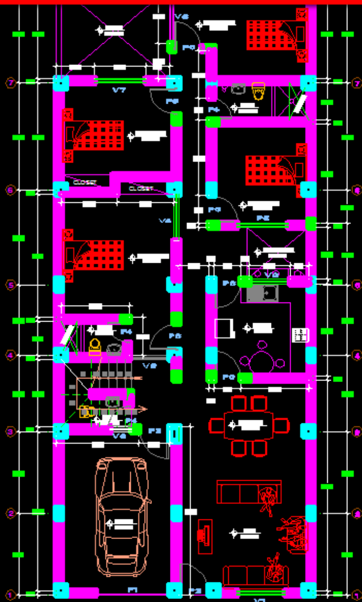
1er NIVEL ESC: 1/50 DISTRIBUCION
