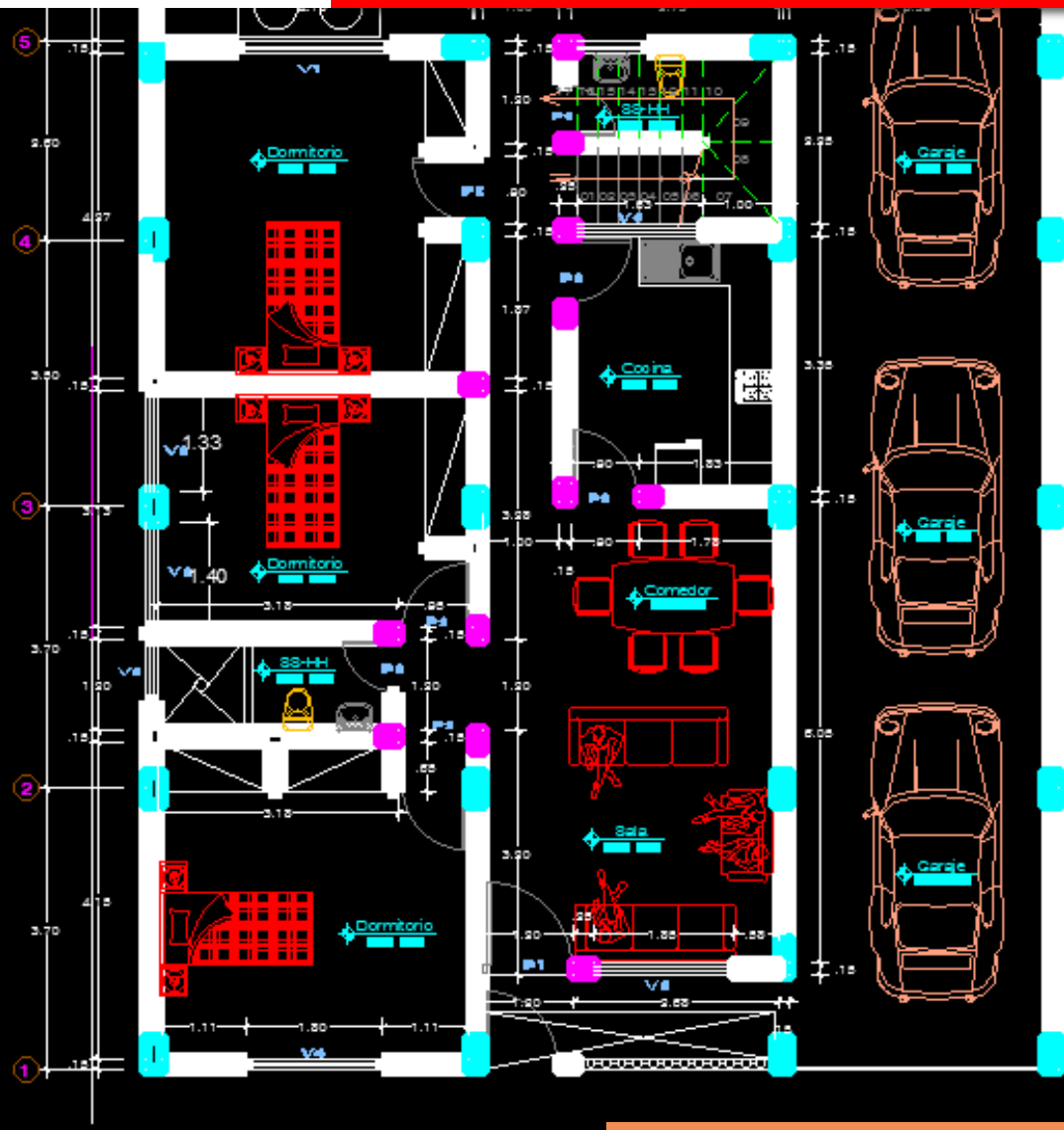
1º NIVEL ESC: 1/50
