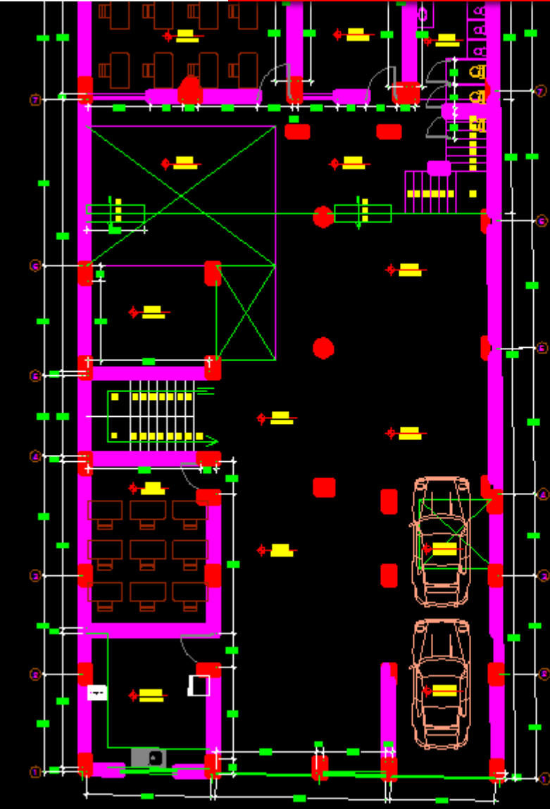
1° PISO DISTRIBUCION ESC: 1:50
