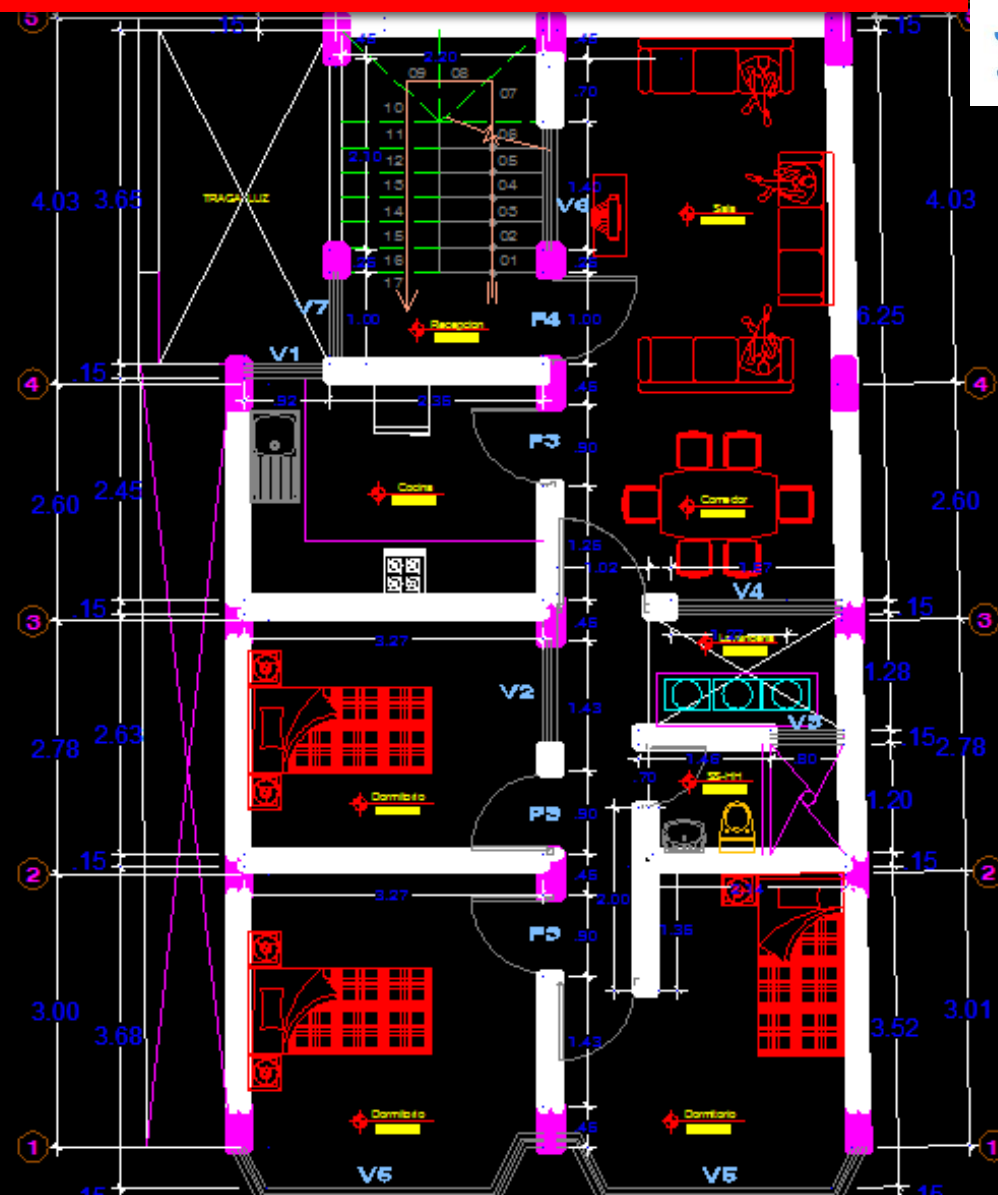
2° NIVEL
