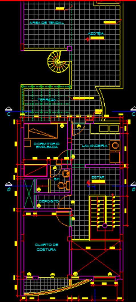
PLANTA: TERCER PISO
