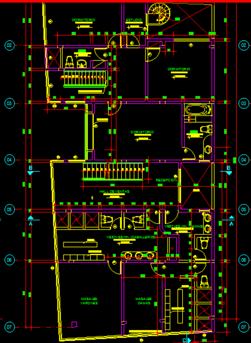
SEGUNDO PISO
