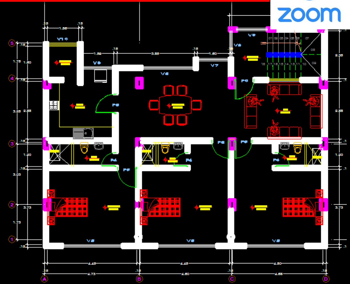
2° NIVEL Asotea E.S.C. 1:50
