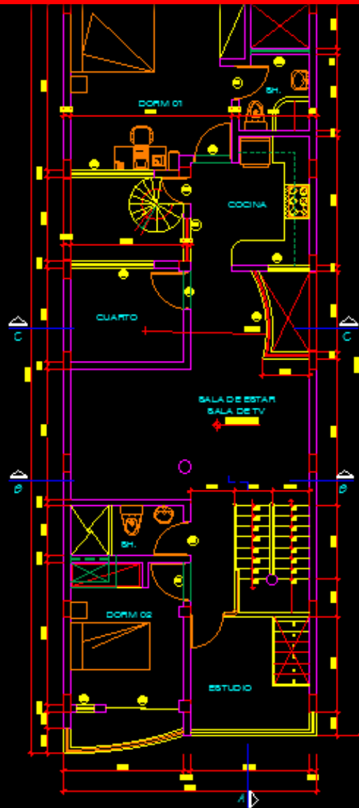
PLANTA: SEGUNDO PISO ESC. 1/50
